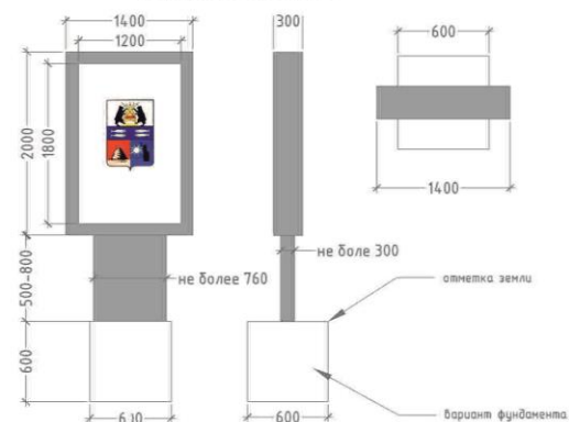
Вариант конструкции
