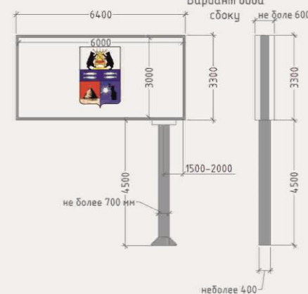
Вариант вида сбоку
